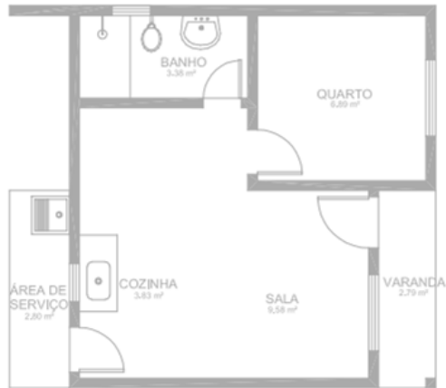
Figura 10: Projeto tipo 3. Fonte: Fundação Prefeito Faria Lima - CEPAM
