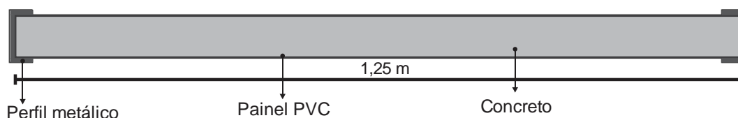
Figura 15: módulo concreto PVC e Steel Frame
