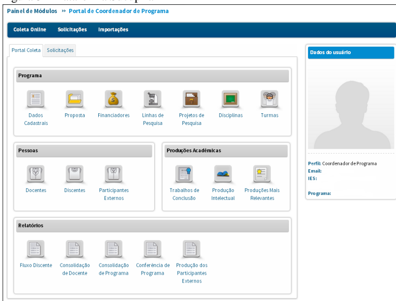
Figura 3 - Plataforma Sucupira
