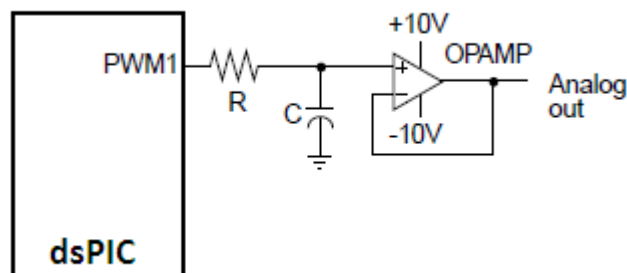
Figura 33. Filtro paso bajo conectado al canal 1 del módulo PWM.
