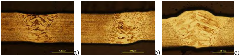
1. ábra. Hozaganyag hozzáadásának hatása a varrat alakra 2205/1,5mm mintasorozatonál. Marószers:Kalling'2 reagens N= 25x; v lézersugár = 1500mm/perc a) autogén hegesztés, b) poradagolás 15 g/perc c) huzaladagolás 1000 mm/perc
