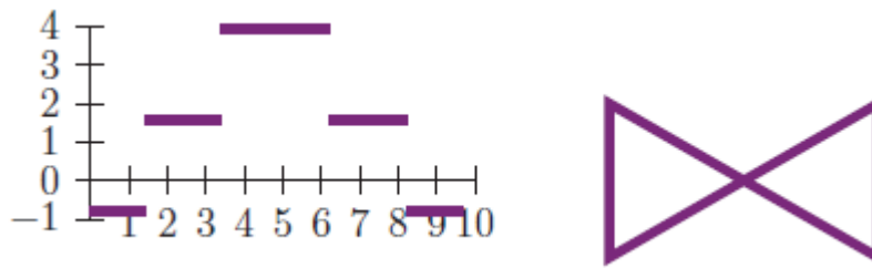
Figura 2. Reconstrucción de un corbatín
