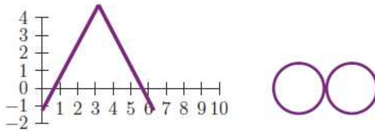
Figura 4. Función angular de un ocho acostado
