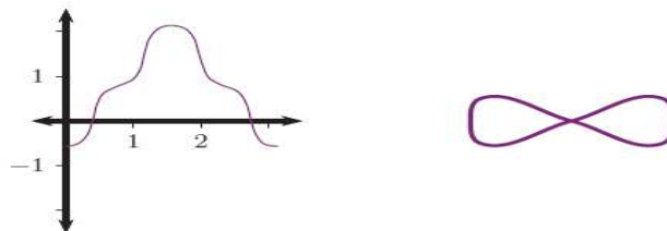
Figura 5. Reconstrucción de una curva de Lissajous
