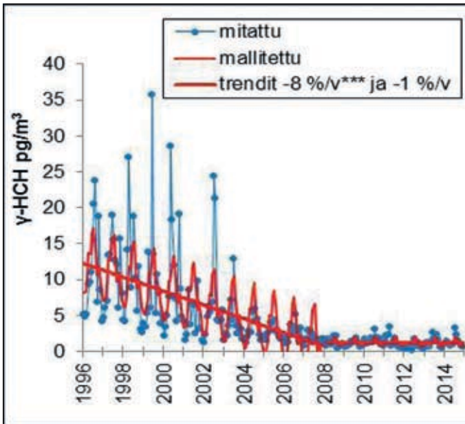
Kuva 1. Kasvinsuojeluaine lindainin ( \gamma -HCH) ilmapitoisuuksien aikakehitys Pallaksella 1996–2014. Vuotuinen muutosprosentin merkitsevyys ilmaistaan tähdillä (erittäin merkitsevä *** p < 0.001 ).
