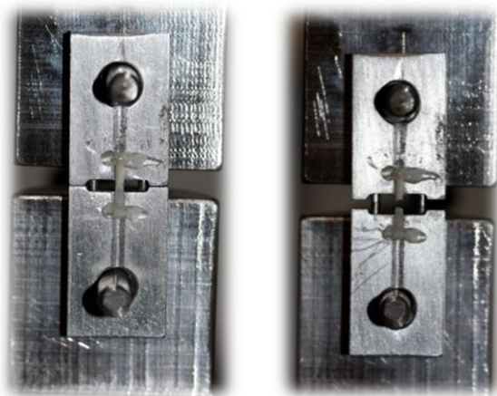
Fig. 25 – Espécimen antes e depois de fraturado após ter sido sujeito a força de tração
