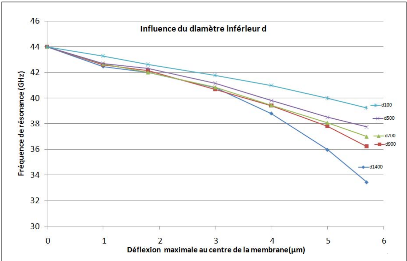
Fig II. 26. Effet du profil de la membrane sur le fonctionnement du capteur EM (pour une membrane d'épaisseur 50\mu\text{m} et une couche d'air de 6\mu\text{m} )
