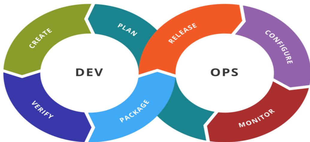
Figura 3.4: Ciclo DevOps
