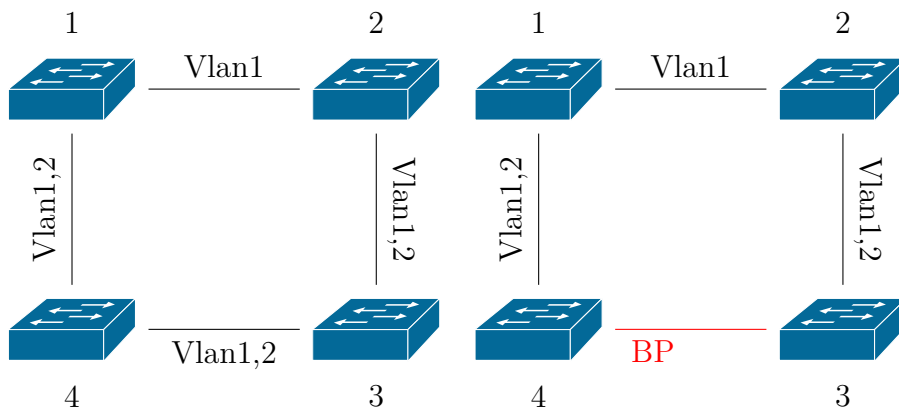
Figura 2.11: Esempio di incompatibilità tra STP e 802.1Q
