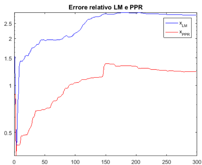
Figura 5.18: Semiconvergenza test 2, rumore 0.1, LM e PPR
