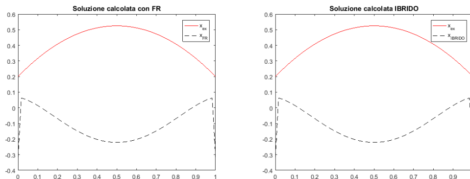
Figura 5.7: Soluzione test 1, FR e IBRIDO , x_0 = \text{ones}(\text{size}(\mathbf{x}_{\text{ex}}))
