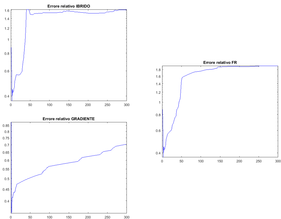
Figura 5.17: Semiconvergenza test 2, rumore 0.1
