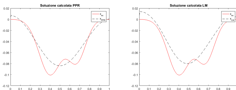
Figura 5.13: Soluzioni test 2, PPR e LM, rumore 0.1, 120 punti
