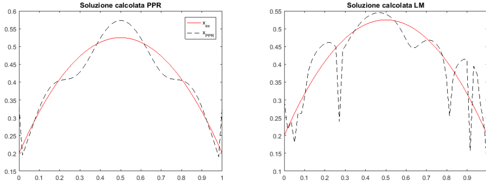
Figura 5.8: Soluzione test 1, PPR e LM, x_0 = \text{ones}(\text{size}(x_{ex}))
