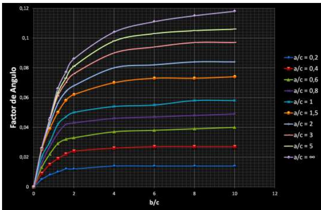
Fig. 4.A: Valor medio del Factor de Ángulo entre una persona sentada y un rectángulo horizontal cuándo la persona es rotada alrededor del eje vertical. Adaptados de la ref. (13)
