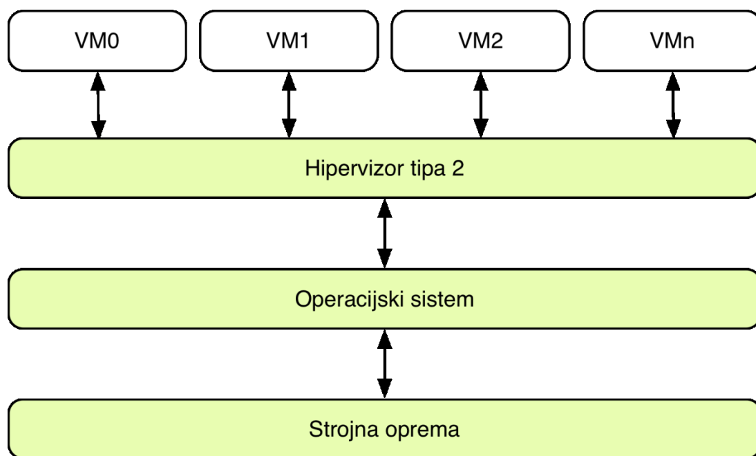
Slika 2: Hipervizor tipa 2
