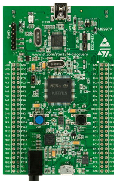
Slika 3.1: Razvojni sistem STM32F4-Discovery
