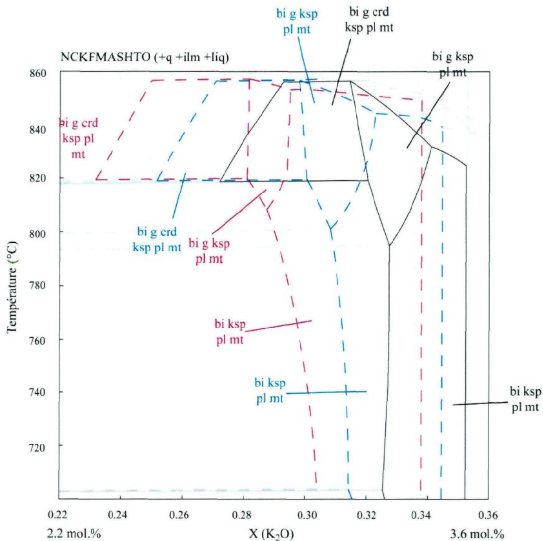
Figure 4.9: Comparaison des champs d'équilibre des diagrammes T-X de SL-75 Ligne noire: T-X(K 2 O) à 1 mol.%H 2 O fixe; ligne bleue: T-X (K 2 O) à 3 mol.%H 2 O fixe ; ligne rouge: T-X(K 2 O) à 5 mol.%H 2 O fixe.
