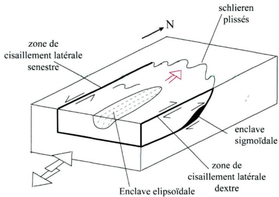
Figure 2.11: structure lobée syn-magmatique dans le granite
