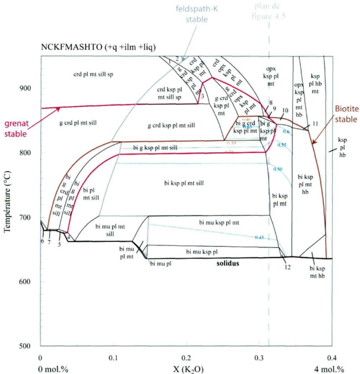
Figure 4.7: Diagramme T-X pour SL-75 à 3 mol.% H 2 O à 6.5 kbar
