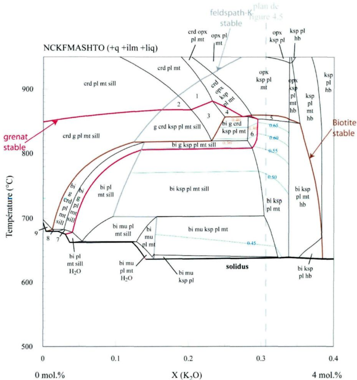
Figure 4.8: Diagramme T-X pour SL-75 à 5 mol.% H 2 O à 6.5 kbar
