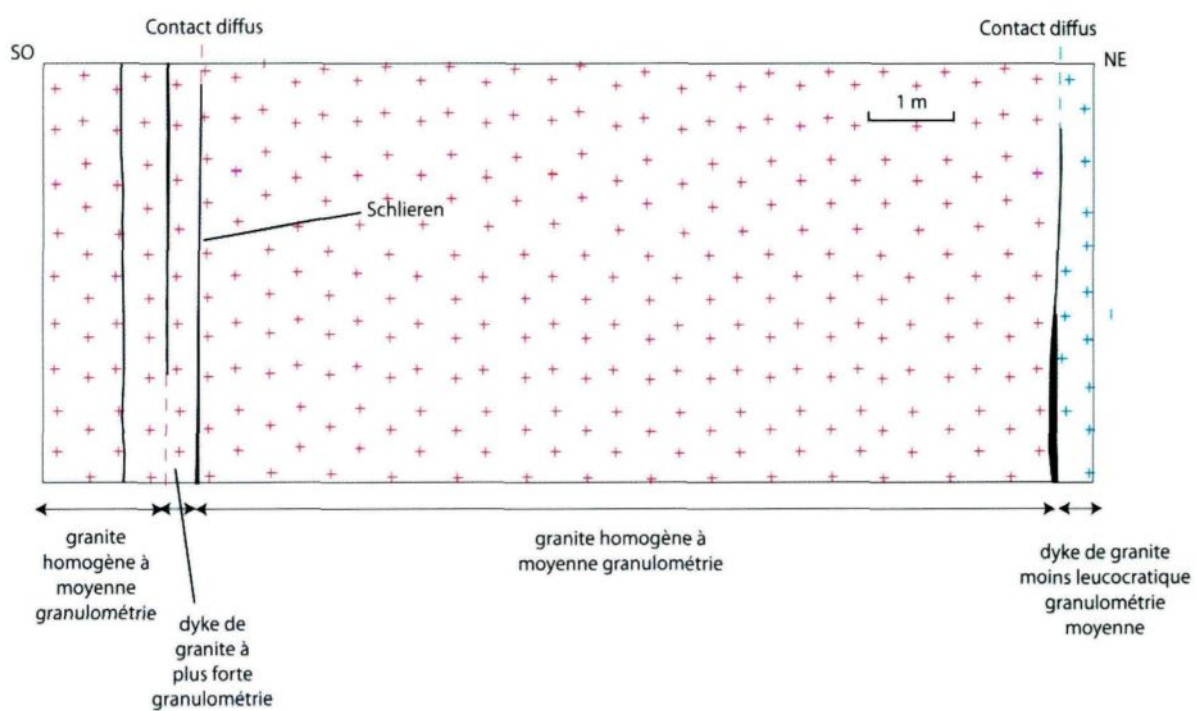
Figure 2.6: Schéma d'affleurement
