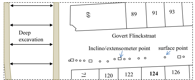
Fig. 15. Top view of deep excavation and buildings Govert Flinkstraat (Ceintuurbaan)
