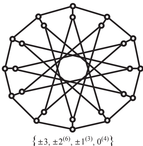
The Nauru 1 graph GP(12,5)
