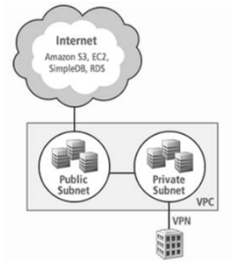
Рис. 3.10. Архітектура гібридної хмари з загальнодоступною та корпоративною під мережами і комплектуючими VPN доступу [258].
