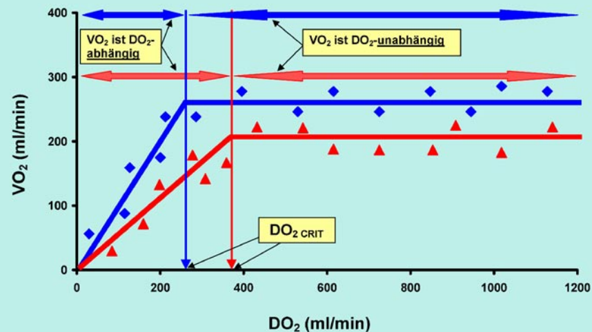
Abb. 2 ▲ VO 2 -DO 2 -Diagramm. VO 2 -DO 2 -Beziehung: Zwei beispielhafte Patienten mit unterschiedlichem Grundumsatz (und somit unterschiedlichem VO 2 -Niveau unter Normalbedingungen) sind dargestellt. Der kritische DO 2 -Wert ist individuell verschieden und abhängig vom Grundumsatz und der individuellen Kompensationsfähigkeit
