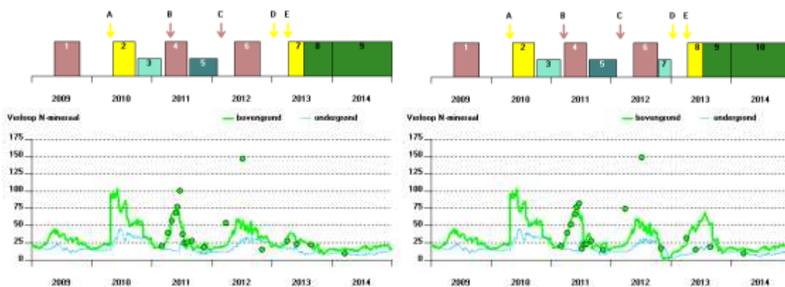
Figuur 4. Vruchtopvolging en verloop van N-mineraalgehalten in de bodem voor perceel 1 A.
