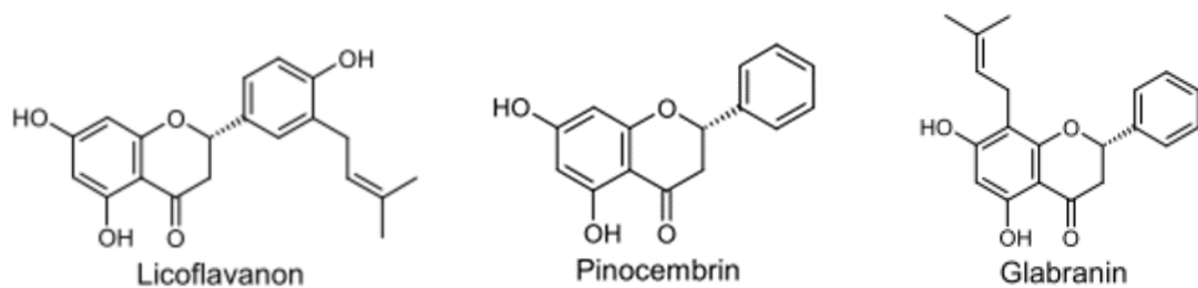
Abb. 4: Strukturformeln der Inhaltsstoffe LPG
