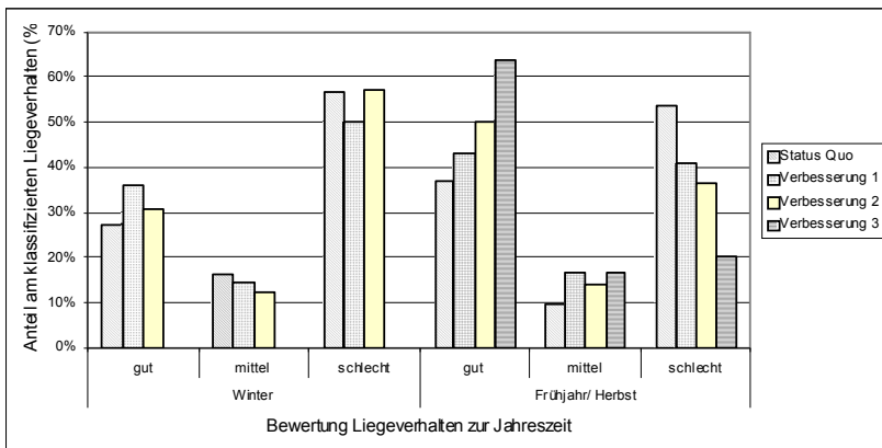
Abbildung 2: Bewertung des Liegeverhaltens mit Einteilung in Werteklassen
