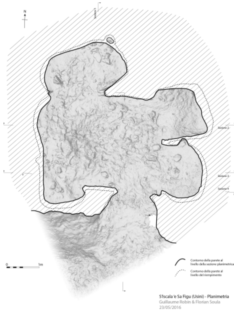
Fig. 10 - Usini. Iscala de Sa Figu. Domus V, planimetria (rilievo G. Robin, F. Soula).
