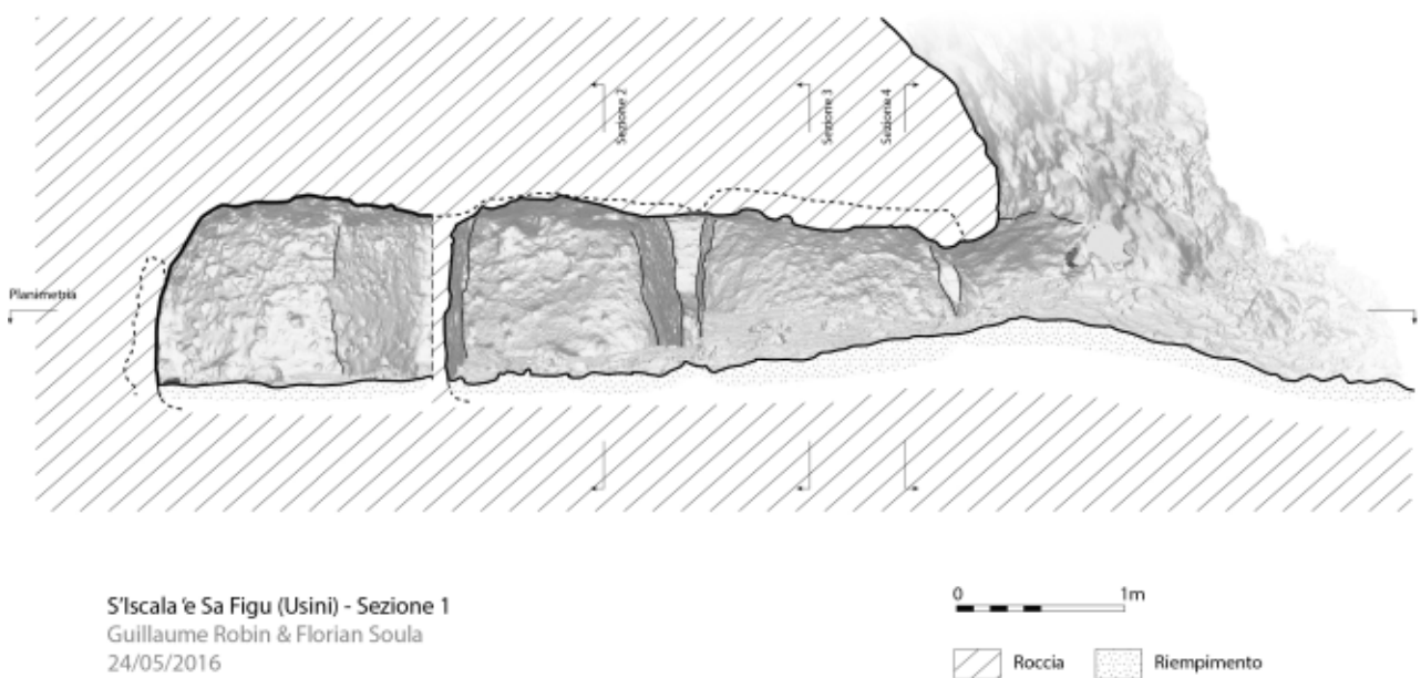
Fig. 11 - Usini. Iscala de Sa Figu. Domus V, sezione I (rilievo G. Robin, F. Soula).
