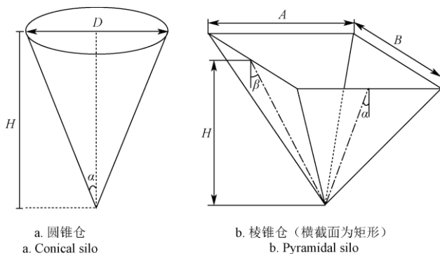
注： \alpha 、 \beta 为锥仓倾角（°），A、B 为仓顶开口内边长（m），H 为锥仓垂直高度（m），D 为仓顶开口内径（m）。 Note: \alpha and \beta are the dip angle（°），A and B are the internal side length（m），H is the height（m），D is the internal diameter（m）.
