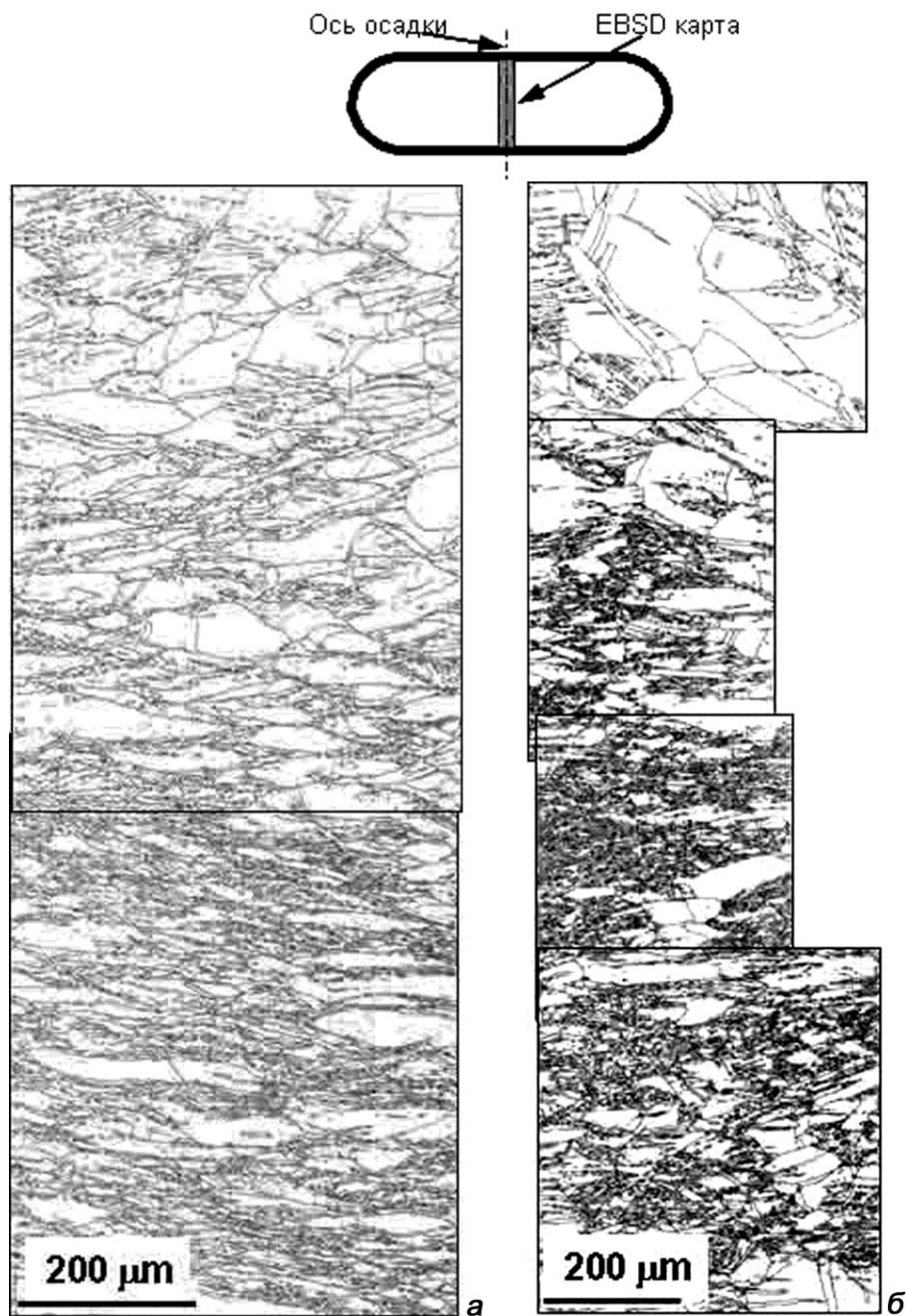
Рис. 2. Изменение микроструктуры по высоте образцов меди, осажденных при комнатной ( а ) и криогенной ( б ) температуре; EBSD-карты (шаг сканирования 1 мкм), показаны только большеугловые границы
