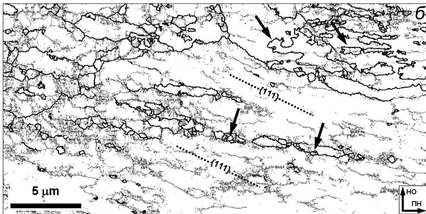
Рис. 4. Микроструктура в центре образцов, осажденных при комнатной (а) и криогенной (б) температуре; фрагменты EBSD-карт (шаг сканирования 0,05 мкм), пунктирные линии соответствуют следам плоскостей \{111\} , стрелками показаны двойники
