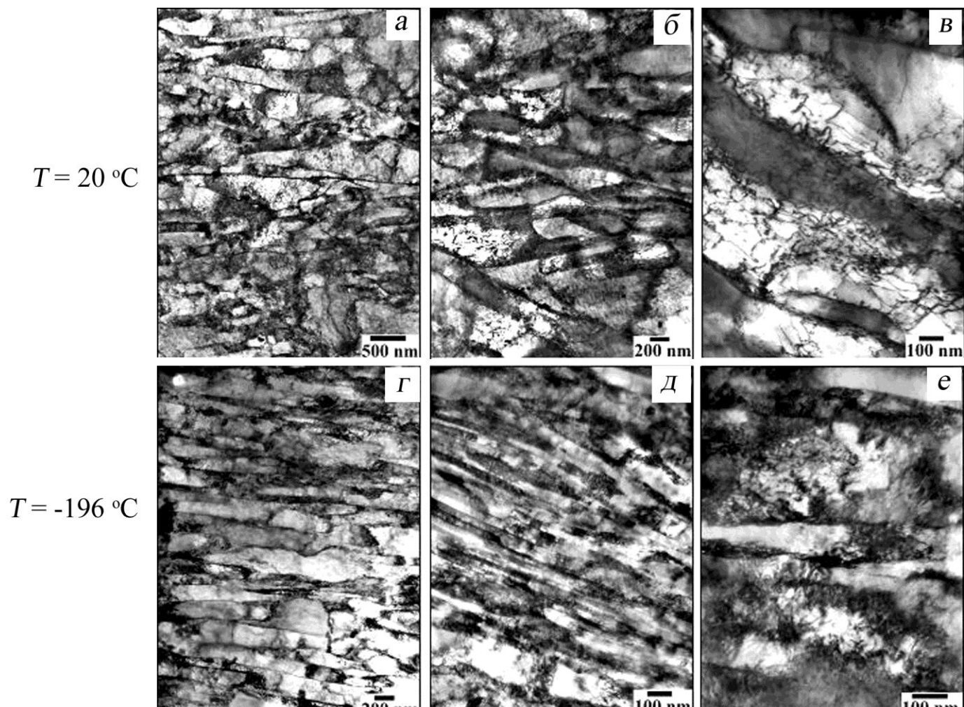
Рис. 6. Тонкая структура после деформации при комнатной ( a–в ) и при криогенной ( г–e ) температуре. Направление осадки вертикальное
