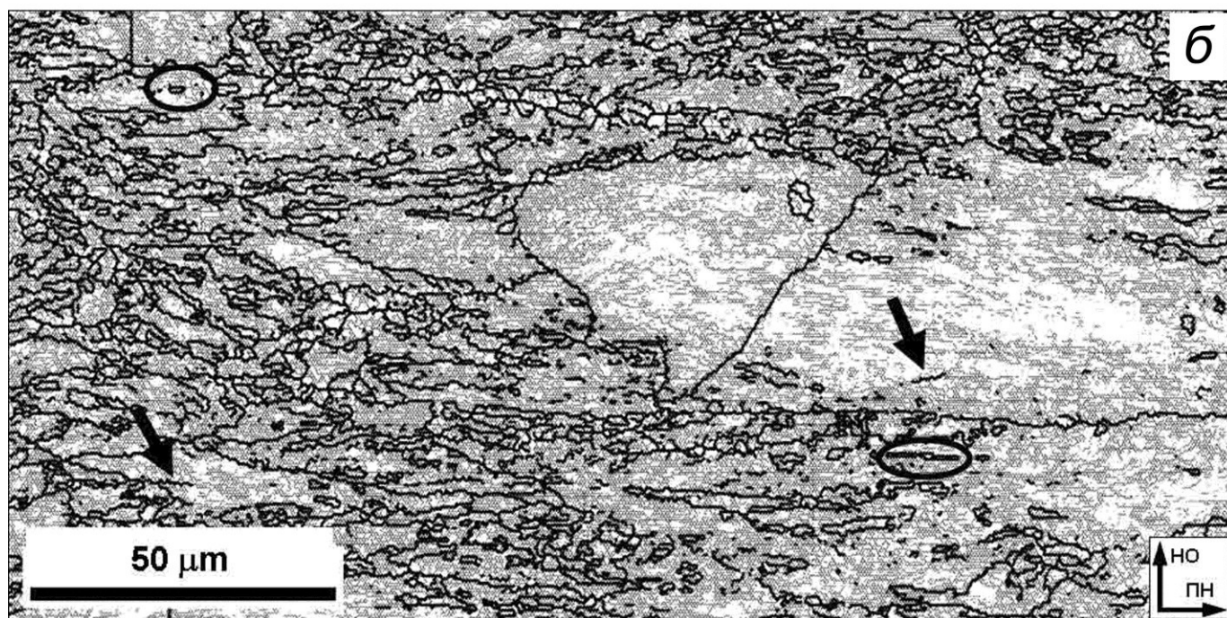
Рис. 3. Микроструктура в центре образцов, осаженных при комнатной (а) и при криогенной (б) температуре; фрагменты EBSD-карт (шаг сканирования 0,5 мкм) МУГ обозначены тонкими серыми линиями, БУГ – толстыми темными линиями, НО – направление осадки, ПН – поперечное направление, стрелками показаны двойники
