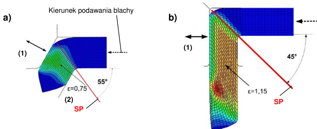
Rys. 1. Rozkład odkształcenia zastępczego \epsilon w przybrzeżnym obszarze blachy po wykonaniu kilku cykli przyrostowego ścinania stemplem (1) działającym w kierunku nieprostym do powierzchni podawanej blachy: a) stempel działający skośnie, b) stempel działający w płaszczyźnie podawanej blachy
