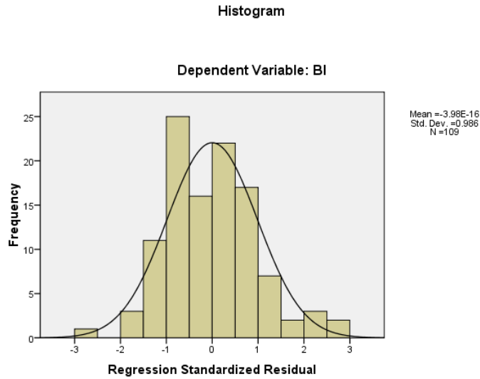
Gambar 4.2 Hasil Uji Normalitas Histogram
