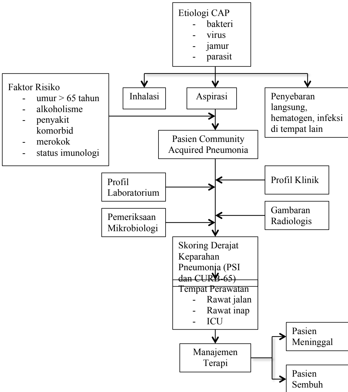
Gambar 2. Kerangka Teori
