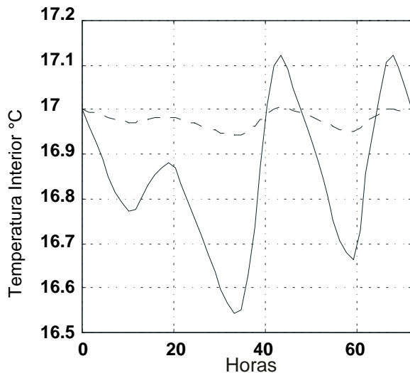
Fig. 1. Temperatura del aire en el invernadero.
