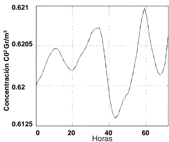
Fig.4. Concentración de CO 2 en ambos modelos.
