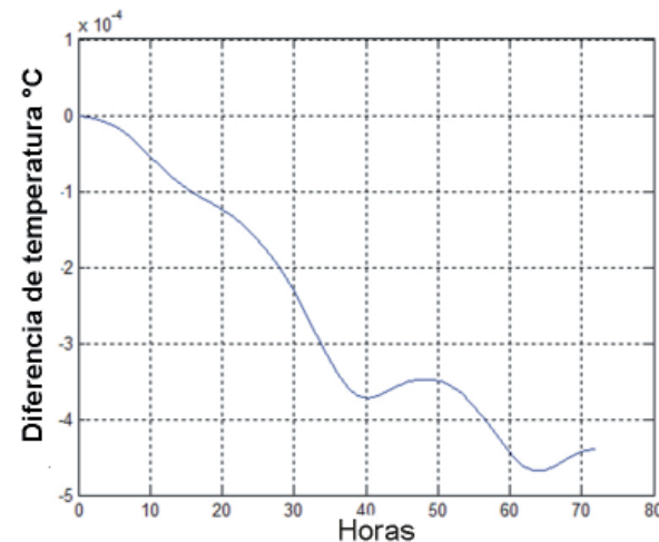
Fig.6. Diferencia de temperaturas del suelo.
