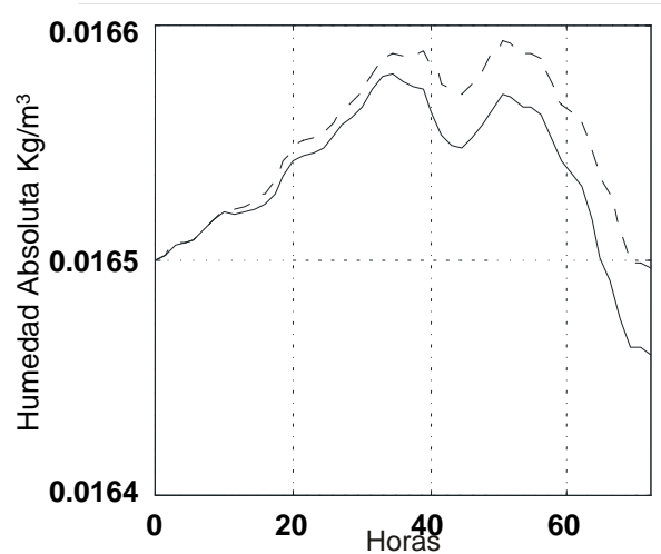
Fig. 2. Humedad en el invernadero.
