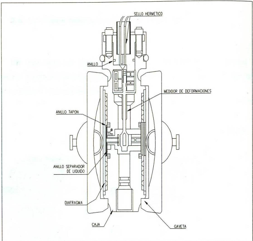
Figura 2.1 Célula Diferencial Tipo "Dri-Flo"
