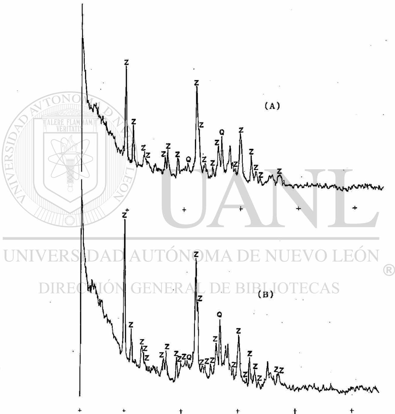
FIGURA No. 4 DIFRACTOGRAMAS DE: A) PUZOLANA NATURAL, Y B) MATERIAL INSOLUBLE DE LA DETERMINACION DE RESIDUO INSOLUBLE.
