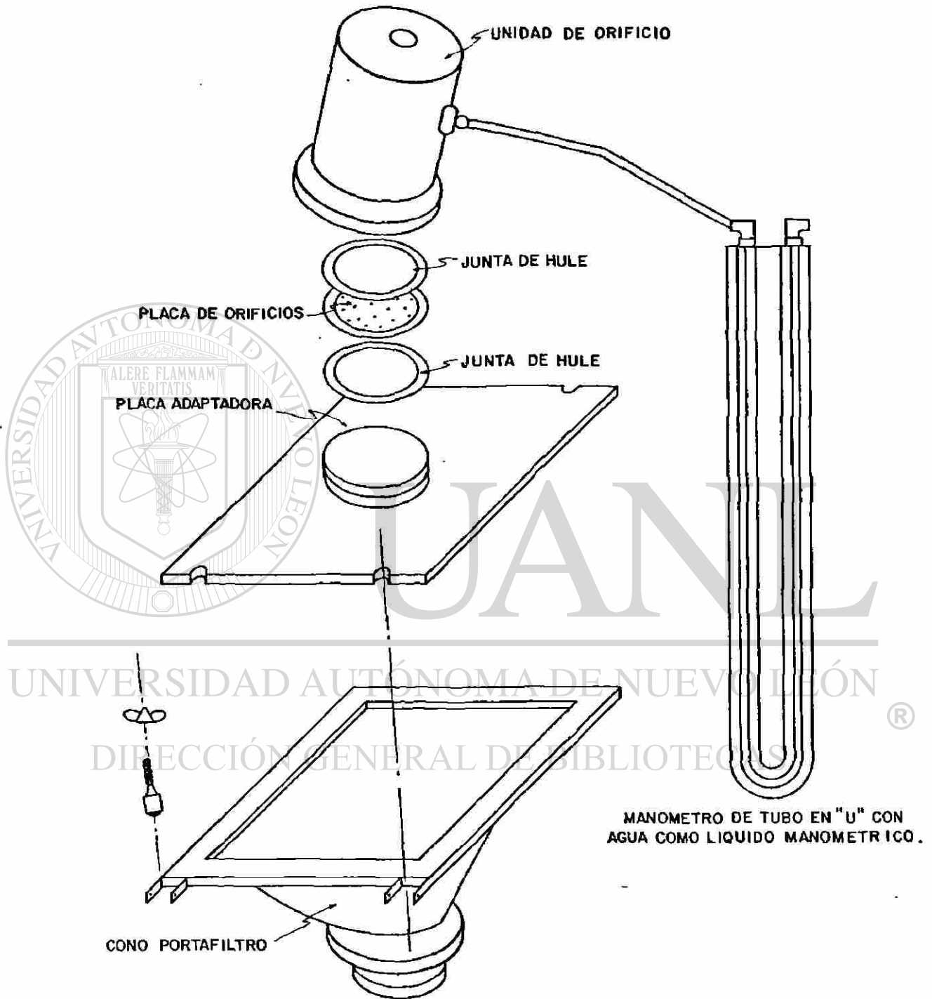
FIG. A-1.3 CONEXION DE LA UNIDAD DE ORIFICIO CON EL CONO PORTAFILTRO, POR MEDIO DE LA PLACA ADAPTADORA.
