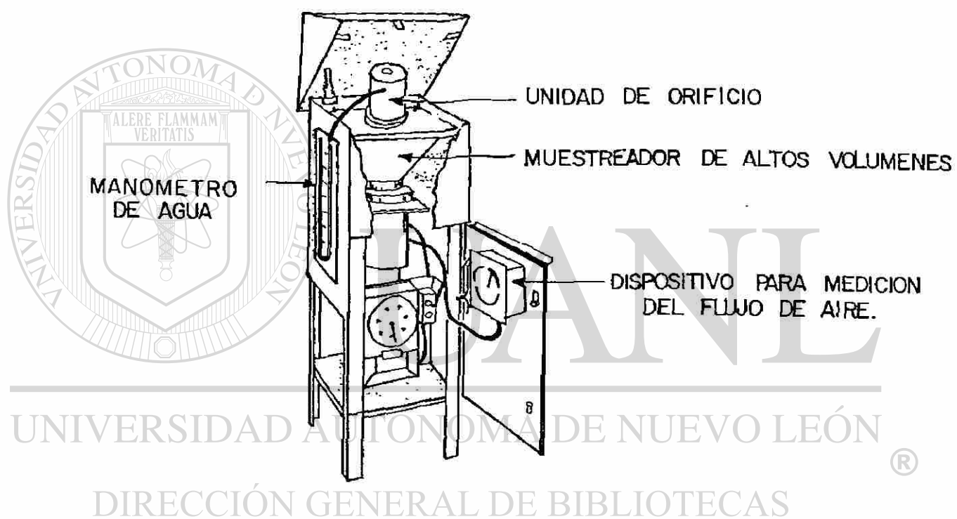
FIG. A.1.1. ARREGLO DEL DISPOSITIVO PARA LA CALIBRACION DEL FLUJO DE AIRE.
