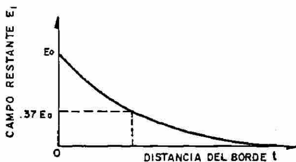
FIG. 1.6 Onda electromagnética atenuada exponencialmente al pasar a través de un medio absorbente.
