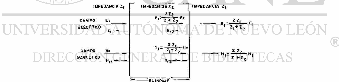
FIG. 1.8 La reflexión y transmisión parcial ocurren a ambas caras del blindaje
