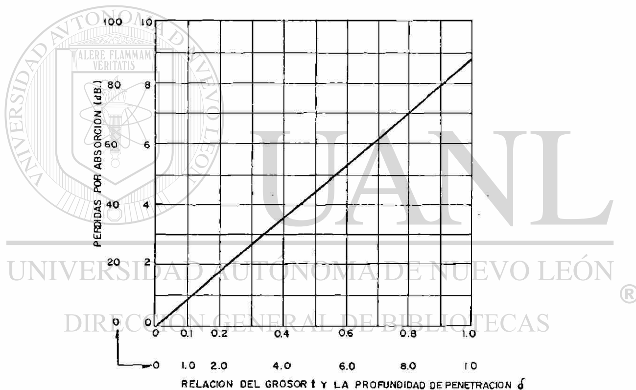
FIG. 1.7 Pérdidas por absorción proporcionales al grosor e inversamente proporcionales a la profundidad de penetración del medio. Para campos eléctricos, campos magnéticos y ondas planas.
