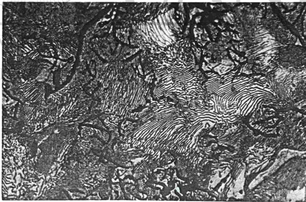
FOT.6.- MICROESTRUCTURA DE OTRA MUESTRA DE MOLDE INGLES. 100x.
