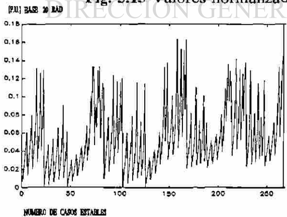
Fig. 5.15 Valores normalizados de diferencia angular. Caso 2.
