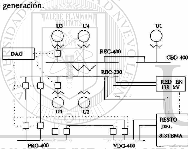
Fig. 4 Esquema del DAG para la planta Río Escondido.
