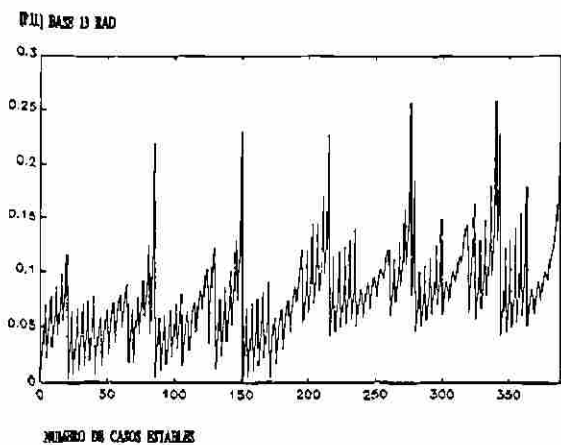
Fig. 5.14 Valores normalizados de diferencia angular. Caso 1.
