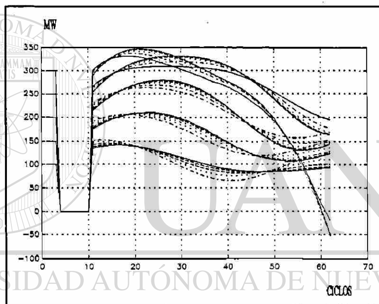
Fig. 3.8 Potencia activa de REC-U2. Caso 1111.
