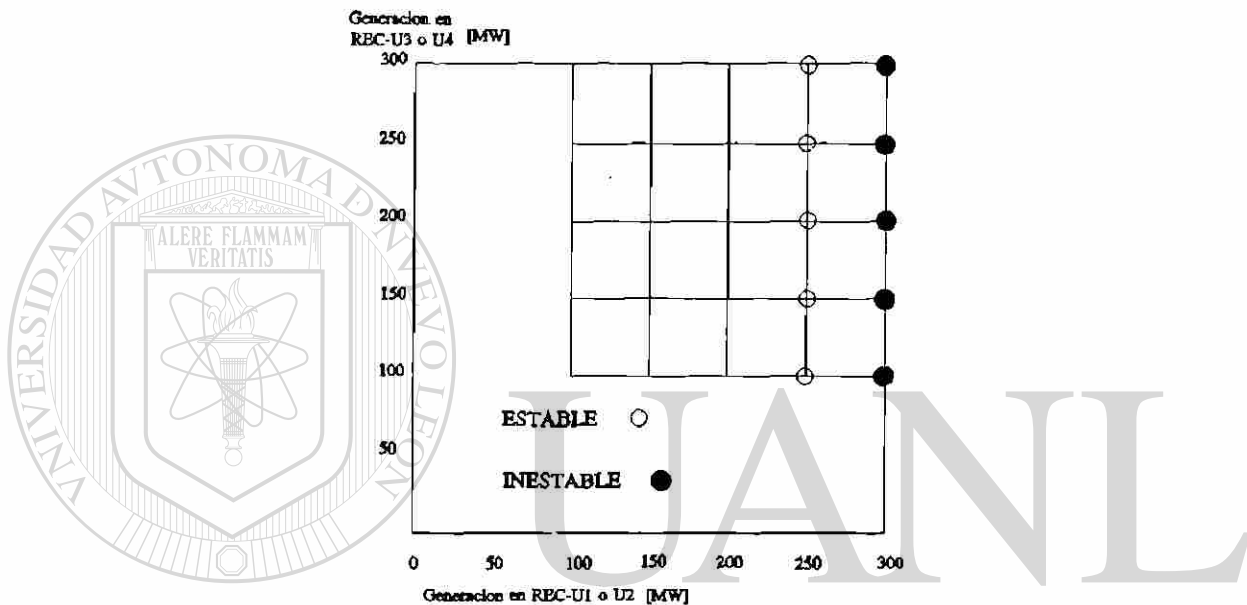
Fig. 3.5 Límites de estabilidad para las unidades conectadas en 230 KV. Caso 1111.
