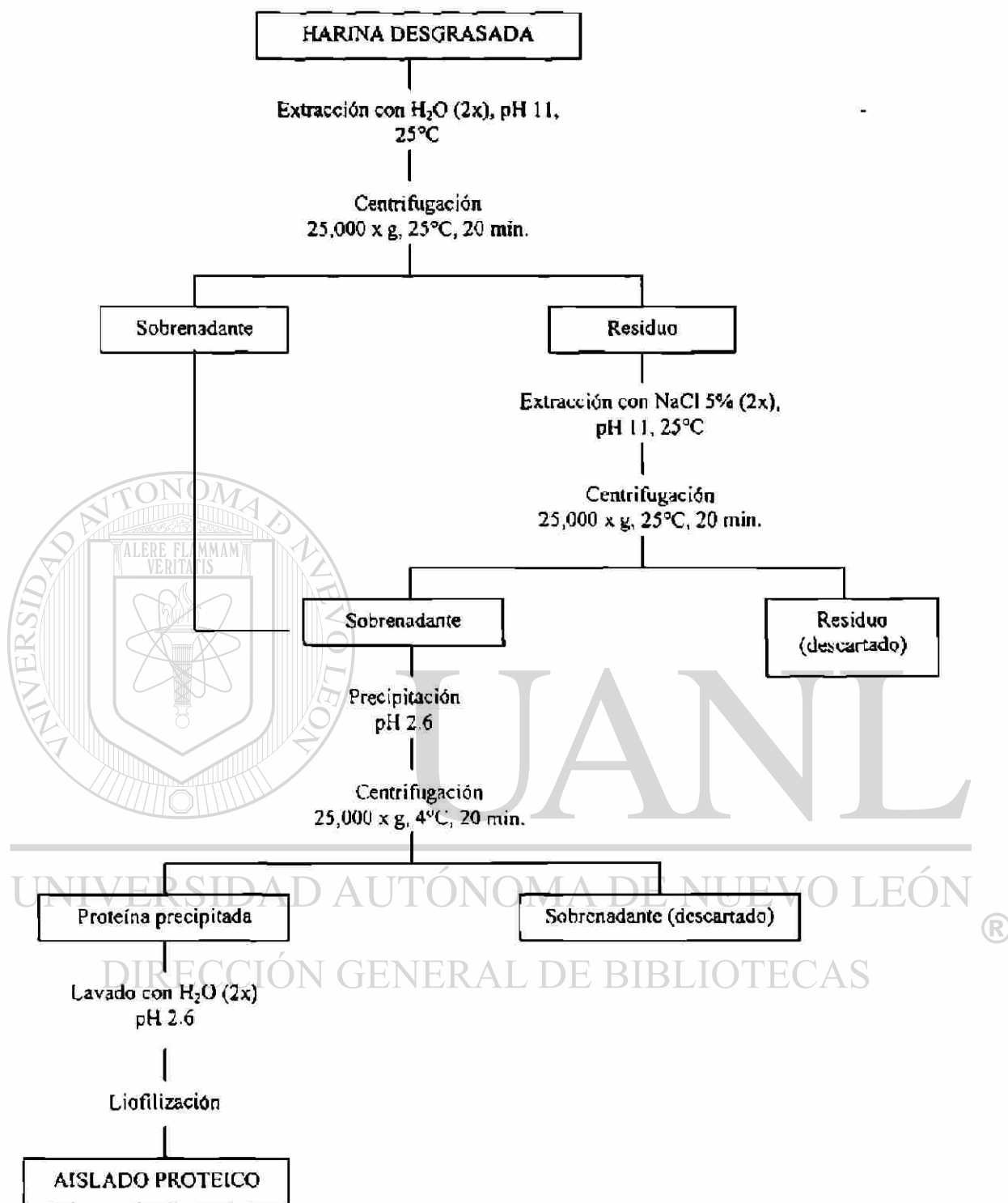
Figura 3.- Diagrama del procedimiento de obtención del aislado proteico de la semilla de ébano. 2x indica que la extracción fue repetida dos veces.
