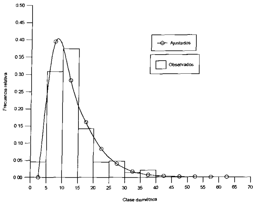
Fig. 5. Ajuste de la distribución Weibull a las estructuras diamétricas (DAP en cm) de árboles de la especie Q. gravesii .
