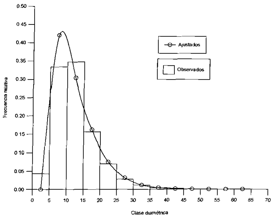
Fig. 4. Ajuste de la distribución Weibull a las estructuras diamétricas (DAP en cm) de árboles de la especie Q. hypoleucoides .
