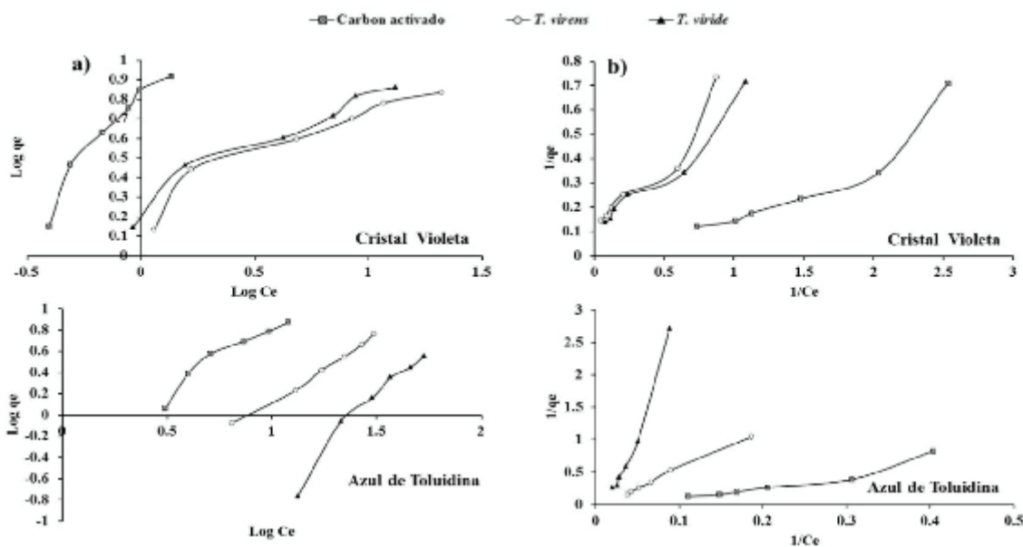
Figura 2. Isotermas de adsorción para Cristal Violeta y Azul de Toluidina por carbón activado y la biomasa seca de T. virens y T. viride a 25°C y pH=6, a) Freundlich y b) Langmuir.
