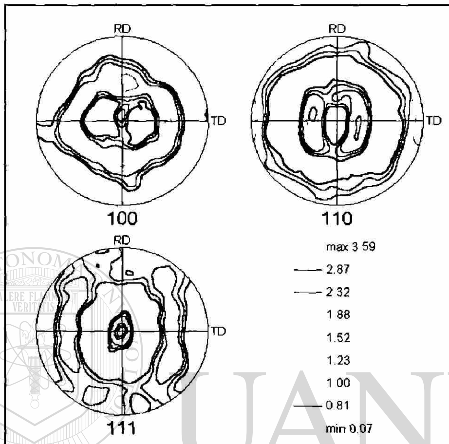
Figura 14. Figura de Polos de una muestra de acero de bajo carbono laminada en caliente 43 .
