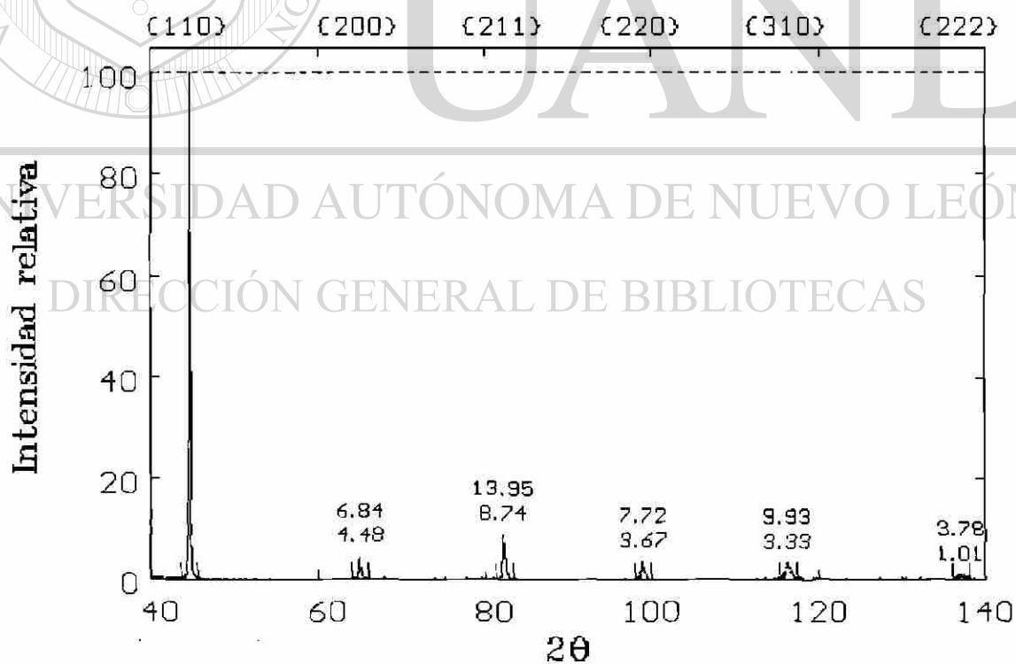
A22. Espectro obtenido a partir de la difracción de rayos X de la muestra B en la zona con deformación.
