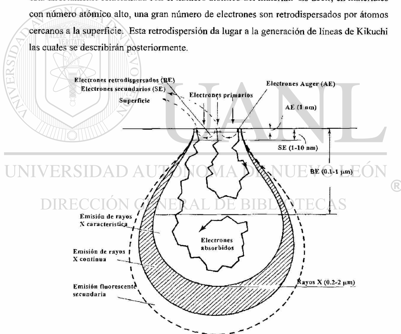
Figura 17. Interacción entre el rayo de electrones primarios y la muestra.
