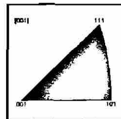
Figura 56, Mapas de distribución de direcciones cristalinicas normales al plano cristalinico de cada grano paralelo al plano de laminación de muestra A3 en la zona sin deformación
