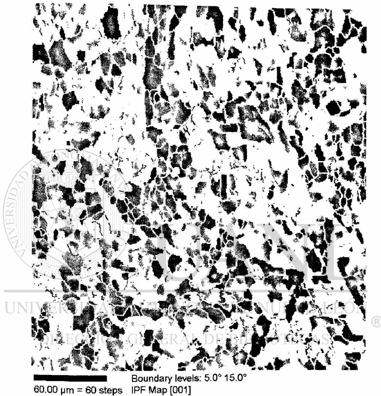
Figura 56, Mapas de distribución de direcciones cristalinicas normales al plano cristalinico de cada grano paralelo al plano de laminación de muestra A3 en la zona sin deformación
