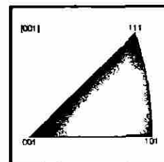
Figura 58, Mapas de distribución de direcciones cristalinicas normales al plano cristalinico de cada grano paralelo al plano de laminación de muestra C en la zona sin deformación
