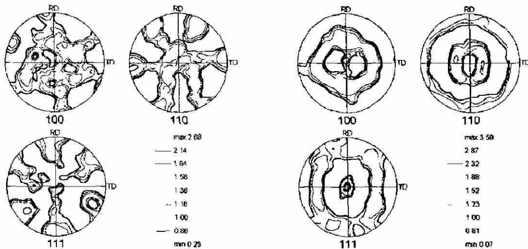
Figura 43. Figura de polos de la muestra A2 deformada del grupo 2.. Figura 44. Figura de polos de la muestra C sin deformación del grupo 2..
