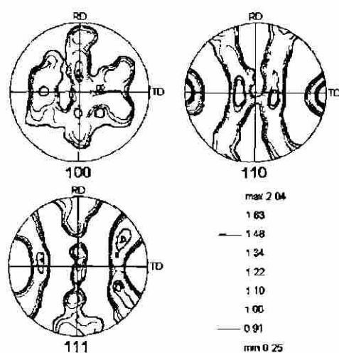
Figura 40. Figura de polos de la muestra A1 con deformación del grupo 2..
