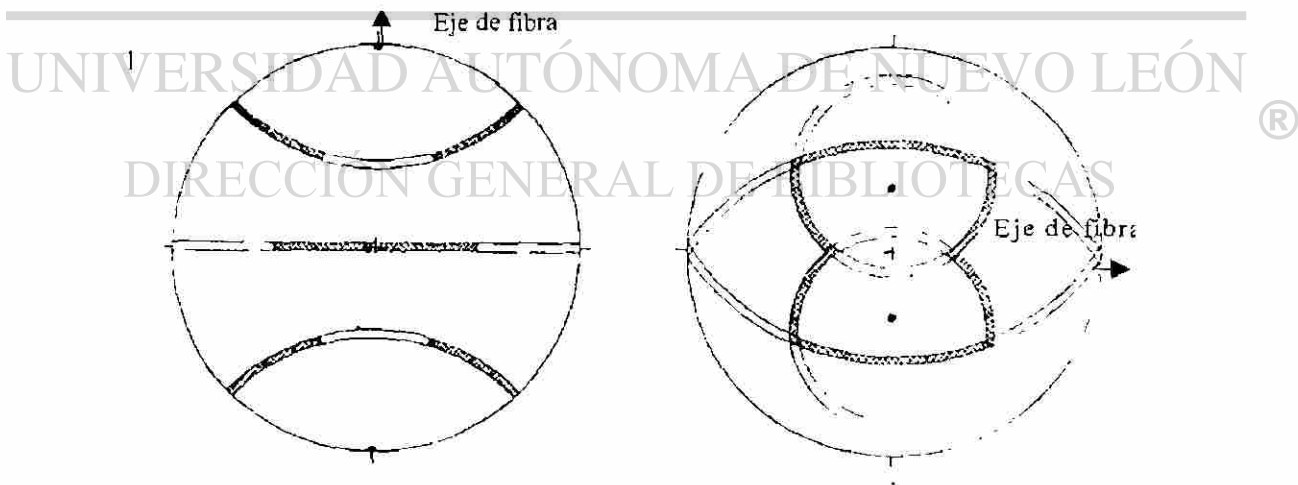
Figura 5. Figuras de polo (100) mostrando la textura de fibra [110] con las dos posiciones del eje de fibra. Las texturas de fibra parciales se muestran en las regiones sombreadas.
