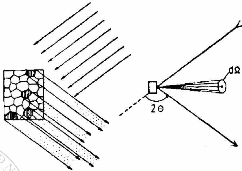
Figura 16. Medición de textura por difracción en policristales.
