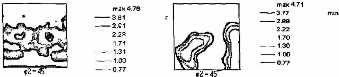
Figura 47. Sección correspondiente a \varphi_2 = 45^\circ de la ODF de la muestra A1 sin deformación del grupo 2..
