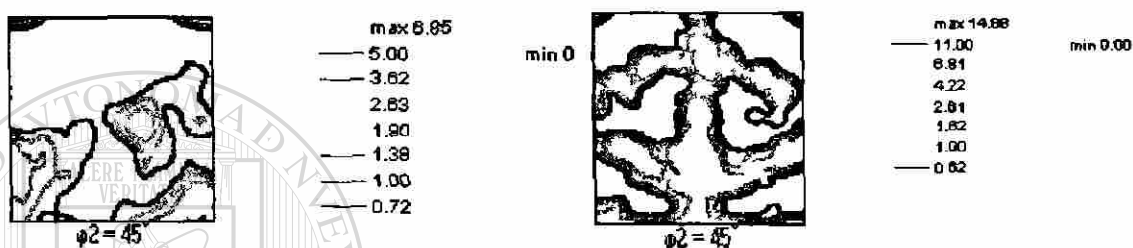
Figura 49. Sección correspondiente a \varphi_2 = 45^\circ de la ODF de la muestra A3 sin deformación del grupo 2..
