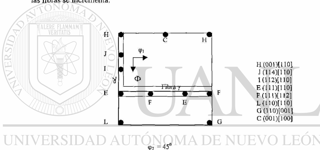
Figura 28. Sección \phi_2 = 45^\circ del espacio Euler. En esta sección se representan las principales orientaciones cristalográficas que se encuentran en las texturas de laminación de materiales bcc.
