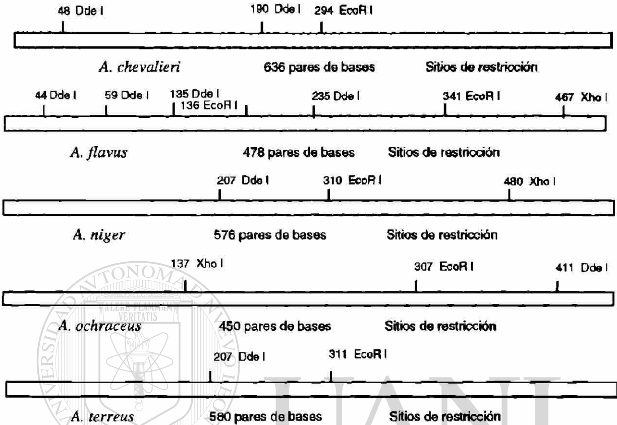
Figura 11. Sitios de restricción de las secuencias ITS en cinco especies de Aspergillus . Sitos generados mediante el programa computacional DNA Strider 1.1.
