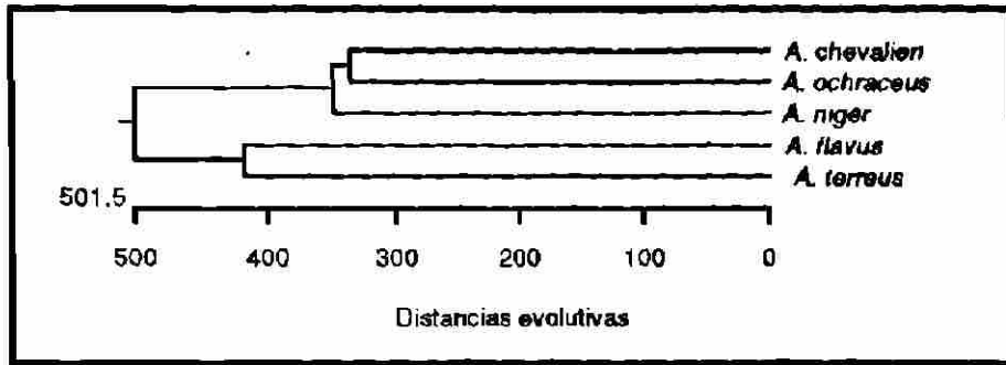
Figura 8. Arbol de las relaciones filogenéticas de las secuencias ITS de cinco especies de Aspergillus . Alineamiento construido con el método J. Hein, el cual se basa en exámenes de pares de secuencias.
