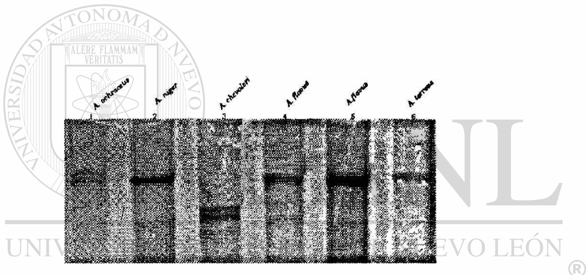
Figura 9. Polimorfismo conformacional de cadena sencilla (SSCP) de los fragmentos ITS de cinco especies de Aspergillus . Electroforesis en gel de poliacrilamida al 6 %. El carril 4 y 5 corresponden a la especie A. flavus , aislamiento nacional y cepa de referencia, respectivamente.
