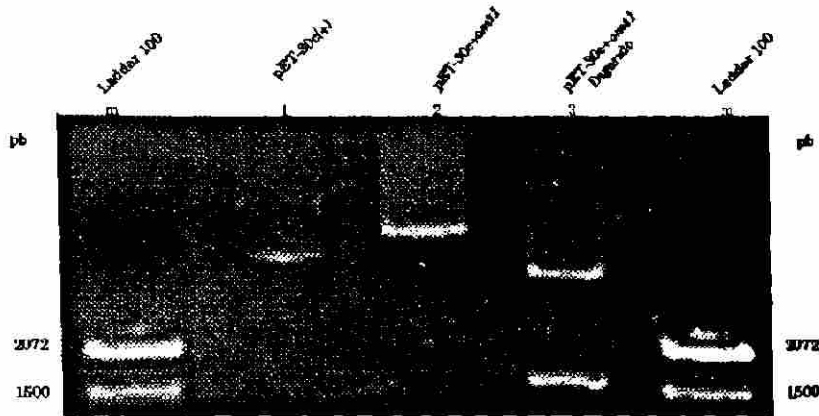
Figura 17. Productos de la digestión enzimática del vector de expresión pET-30c(+). Verificación de la subclonación del gen omt-A en pET-30c(+), mediante la digestión enzimática con Bam H I y Xho I en el carril 3.
