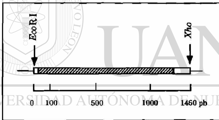
Figura 14. Mapa de restricción del clon omt-A . La región sombreada corresponde al gen omt-A con 1,254 pb y los extremos 5' y 3' están indicados por los espacios en blanco. Tomado de Yu y cols, 1993 (103).
