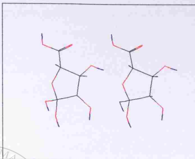
INTERMEDIARIO TETRAHEDRICO DE LA LACTONA DEL AC. L- ARABINARICO (NO SE AISLO)
