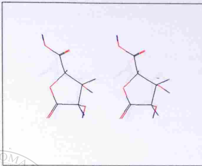
LACTONA DEL ACIDO XILARICO
