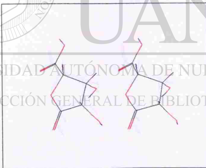
LACTONA DEL ACIDO RIBARICO ESTRUCTURA (3)
