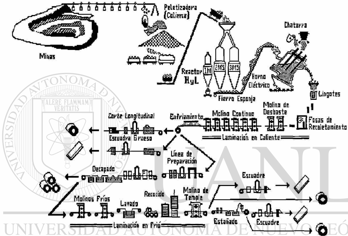
Fig. 2.1: Proceso de obtención de cinta de acero partiendo de la extracción del mineral al producto terminado.
