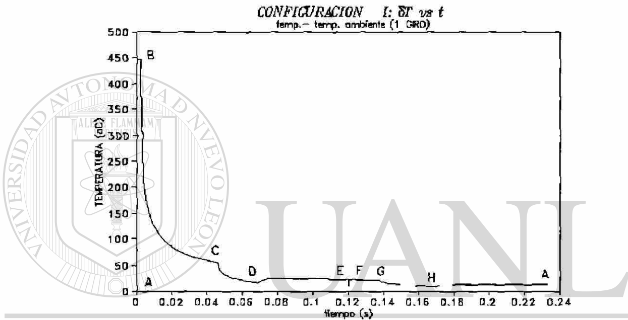
Fig. 6.3: Perfil térmico del primer giro, las regiones de transferencia corresponden a las marcadas en la figura 6.1.
