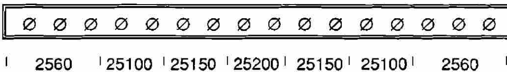
Fig. 5.8: Disposición de las boquillas en los cabezales para los castillos del molino continuo.
