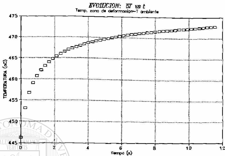
Fig.6.8: Temperaturas correspondientes a la envoltente superior; registradas a la salida de la zona de deformación para los primeros 50 giros.
