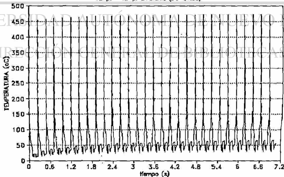
Fig. 7.7: Perfil de temperatura para los primeros 30 giros (configuración II). Nótese el incremento de la temperatura a la entrada y salida de la zona de deformación.
