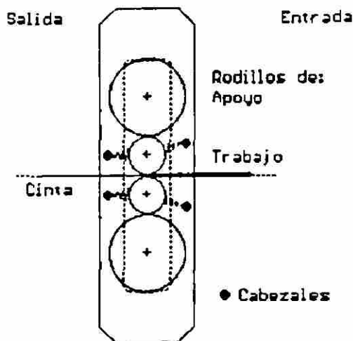
Castillo de laminación
