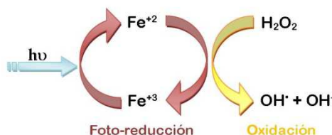
Figura 1. Mecanismo simplificado de los sistemas foto-Fenton
