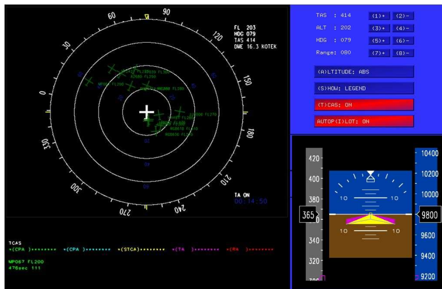
Figura 5: visualizador CDTI
