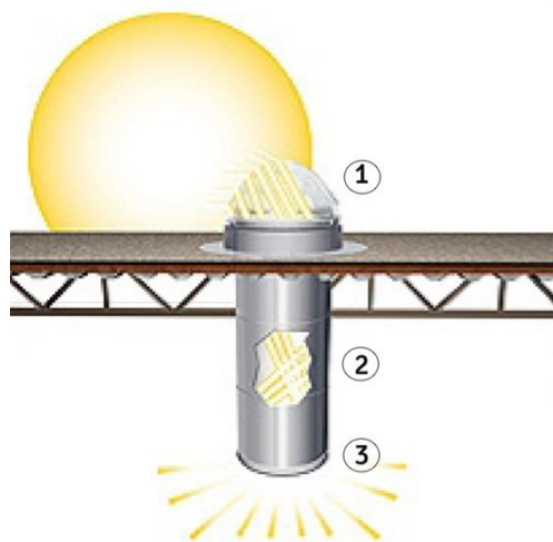
Figura 78: Componentes de un lumiducto
