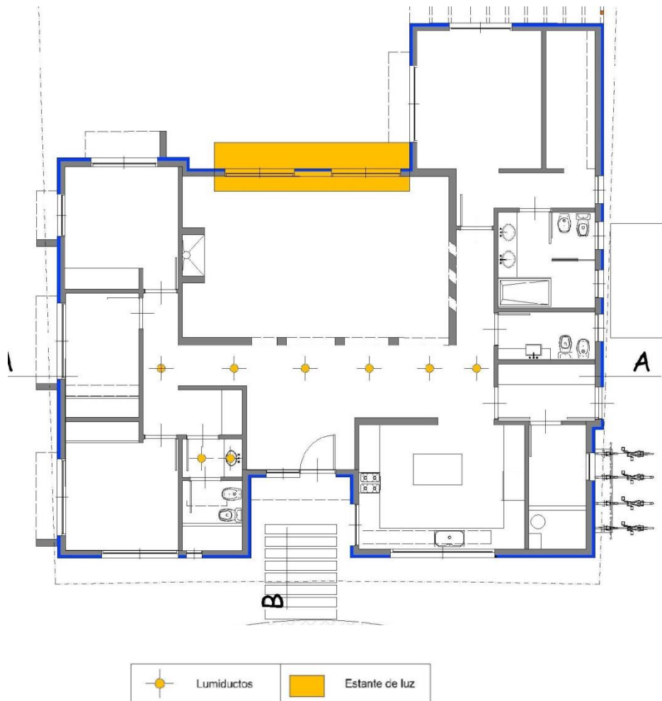
Figura 76 : Planta ubicación de estrategias de iluminación natural.
