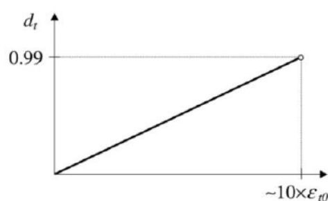
Figura 2: Evolución de la variable de daño.
