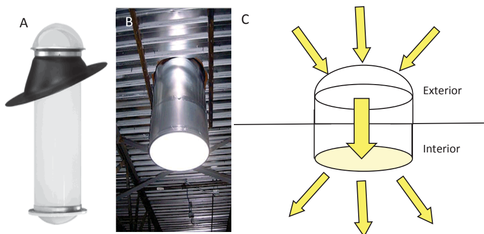
Figura 5. Tubos para luz cenital A) Modelo para techo a dos aguas. B) Para techo plano. C) Esquema del funcionamiento del difusor de luz desde el exterior hacia el interior del ambiente.
