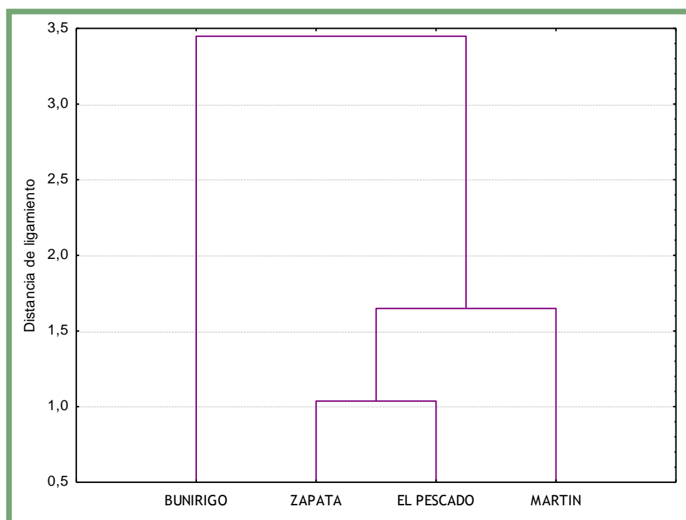
Fig. 2.8. Análisis de Clusters realizado en base a los valores medios calculados de los índices bióticos en los sitios estudiados de los cuatro arroyos.
