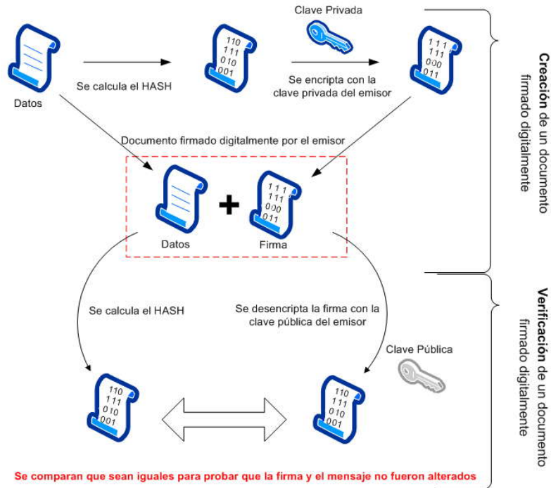
Figura 1: Proceso de Firmado y verificación
