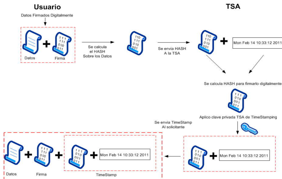
Figura 2: Proceso de Firmado con Time-Stamping
