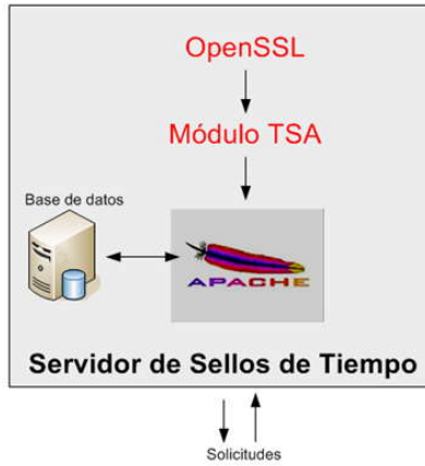
Figura 3: Esquema de funcionamiento de una TSA con OpenTSA
