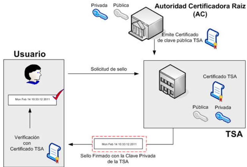
Figura 4: Esquema de funcionamiento de una TSA con OpenTSA
