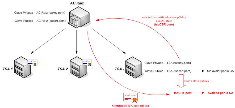
Figura 8: Proceso de generación de certificados
