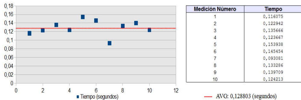
Figura 6: Medición de tiempos de Respuesta-Rafaela
