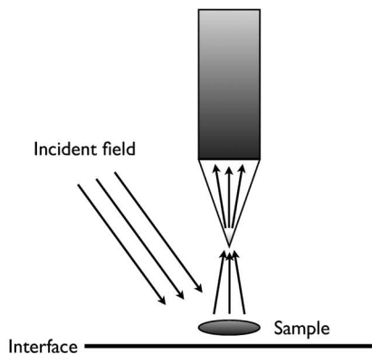
(a) Collection mode NSOT
